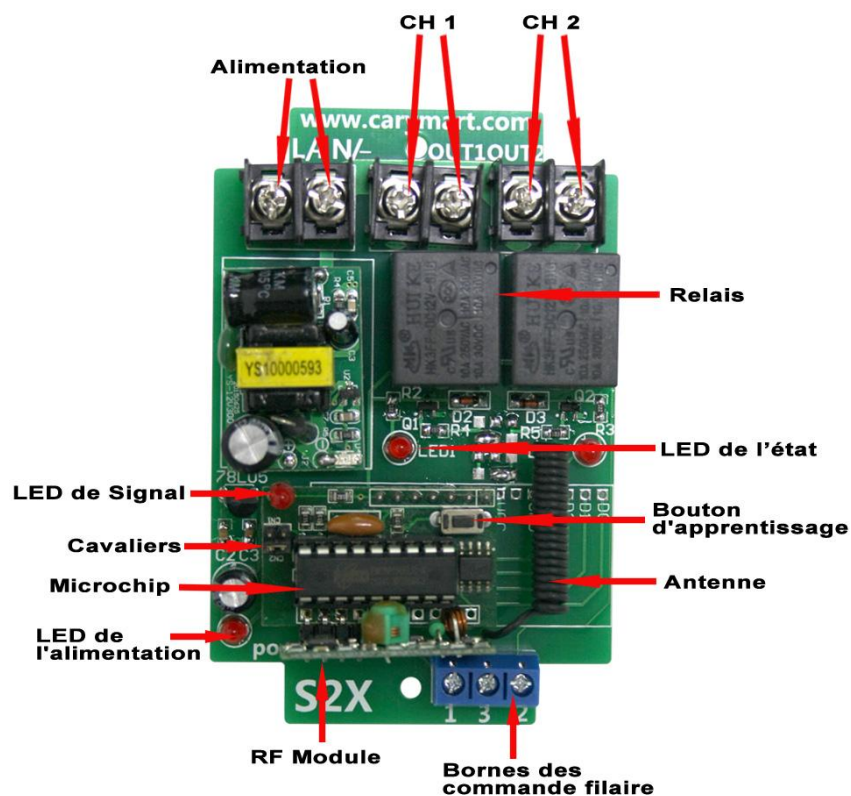
Control moteur CA
