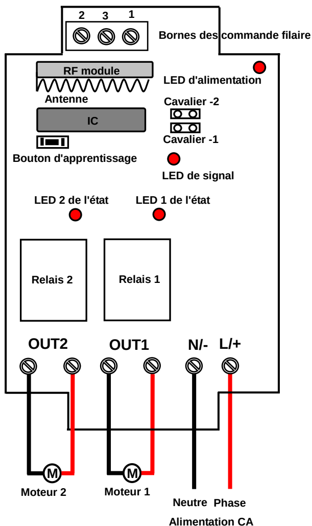
Control moteur CA
