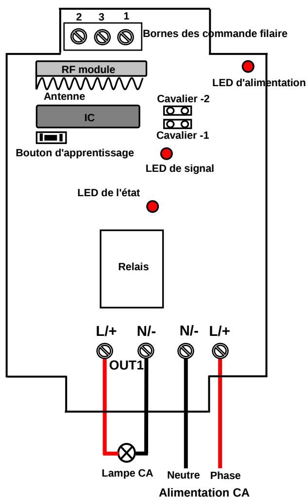
Contrôler lampe CA
