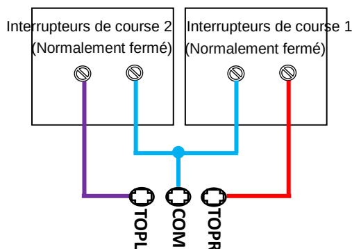
Connecter les Interrupteurs de course
