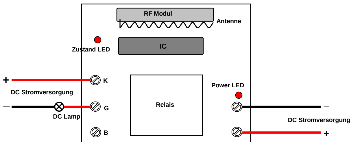
Kontrolle DC Licht
