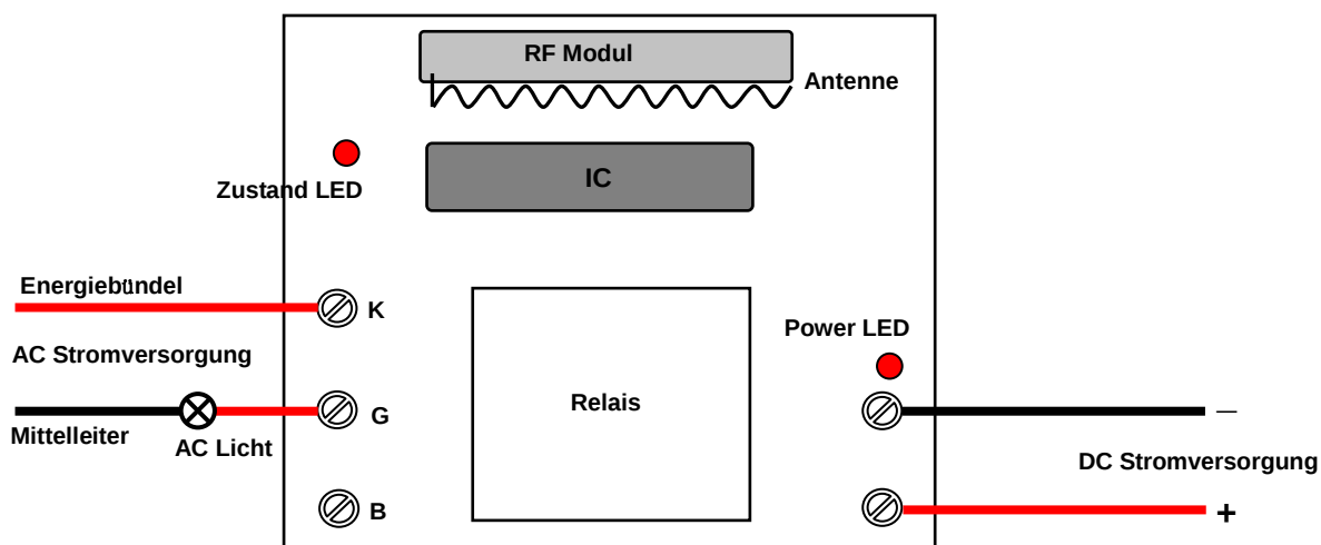
Kontrolle AC Licht
